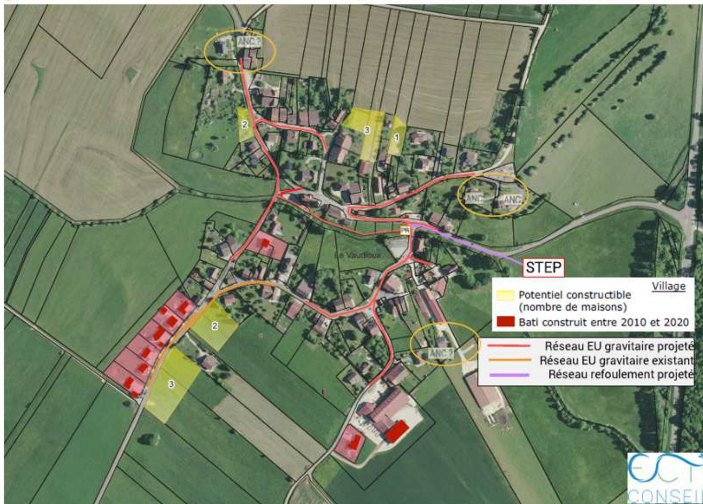
Bourg du Vaudioux - Plan schématique du programme de travaux du scénario 1
