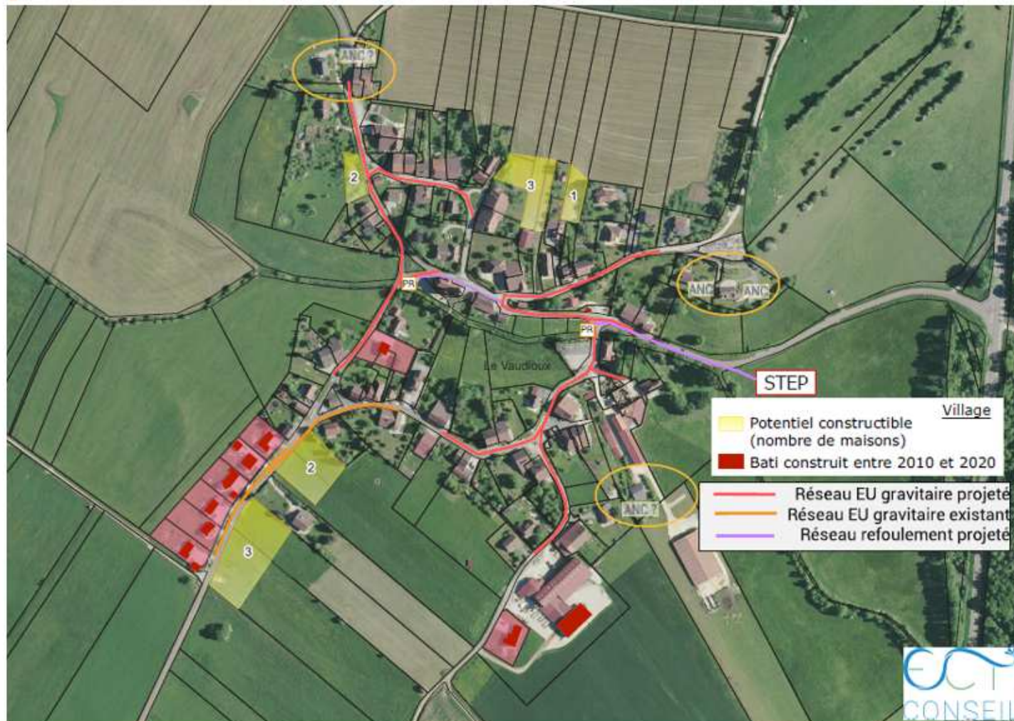
Bourg du Vaudioux - Plan schématique du programme de travaux du scénario 2
