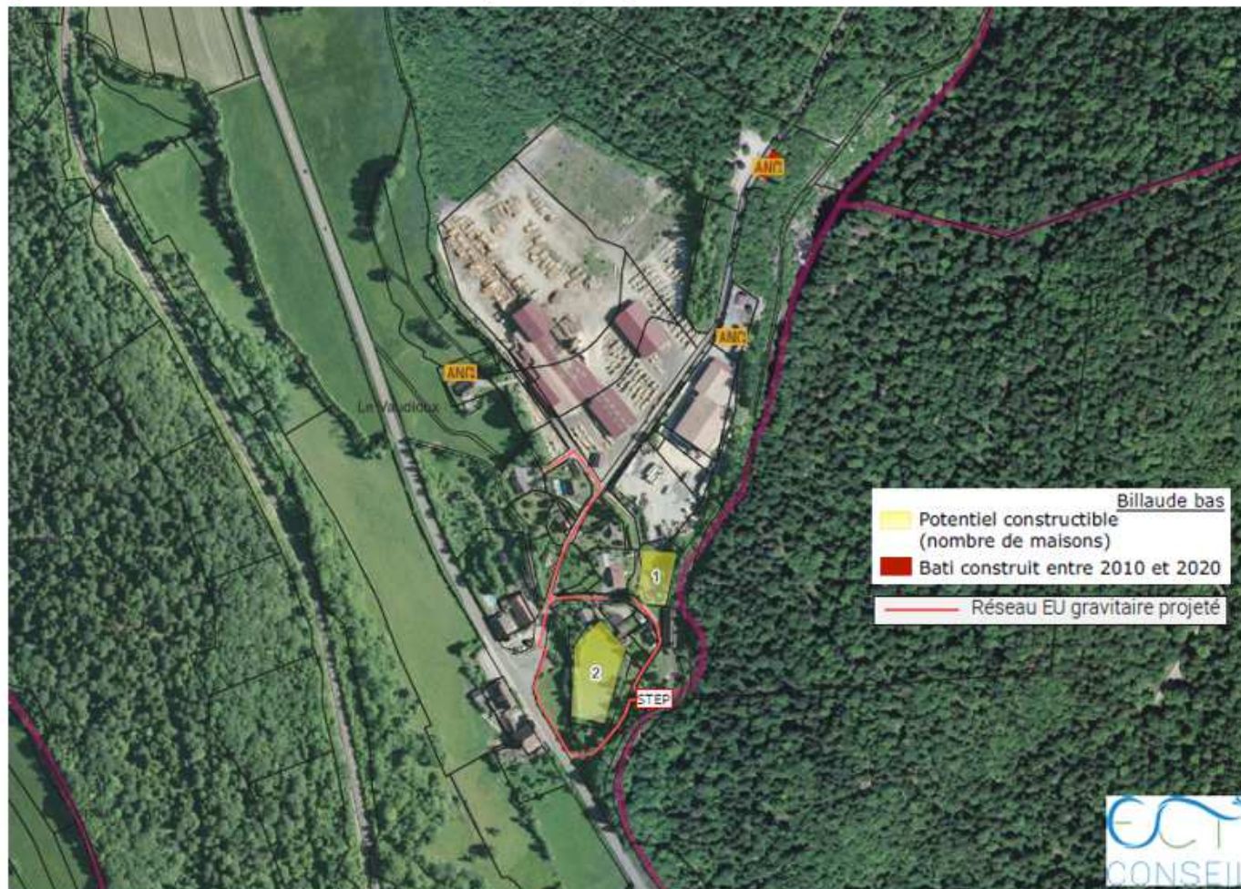
Billaude du Bas - Plan schématique du programme de travaux du scénario 1
